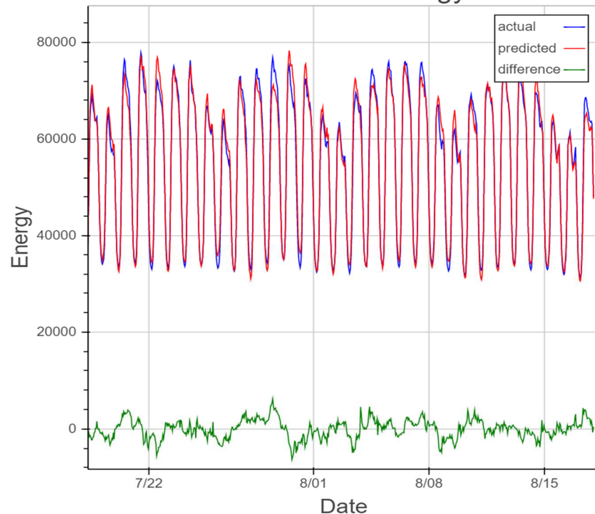
Predicted vs. Actual Energy Use
